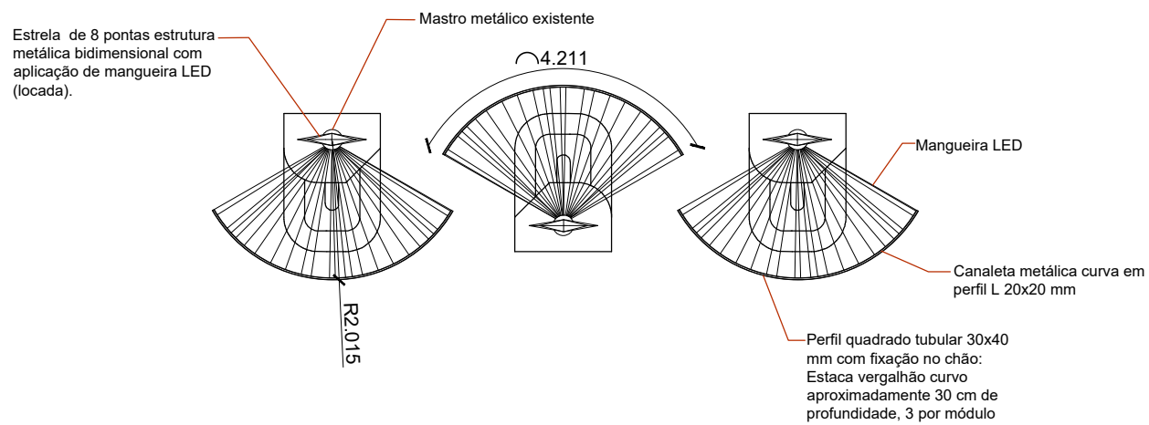
VISTA SUPERIOR ESC. 1:100
