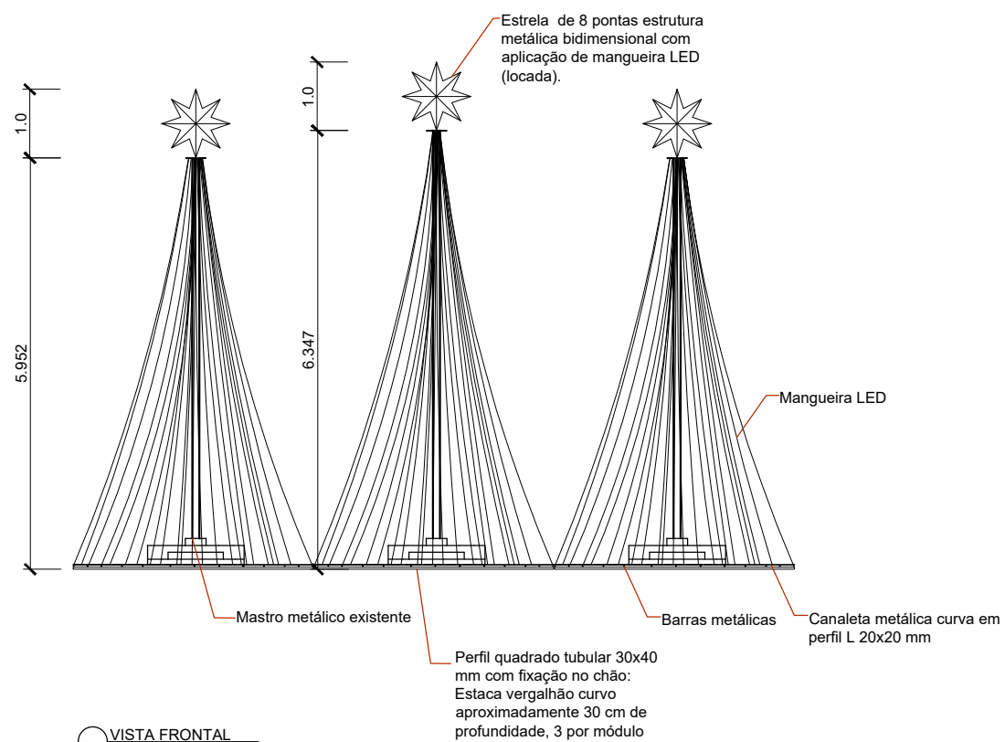
VISTA FRONTAL ESC. 1:100
